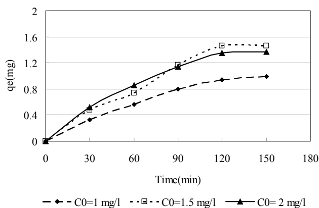
نمودار شماره ۴: تغییرات جذب کروم با زمان در غلظت های مختلف کروم (غلظت کروم ۱/۵ mg/l، دوز جاذب ۰/۷ mg/۱۰۰ ml و pH=۳)
