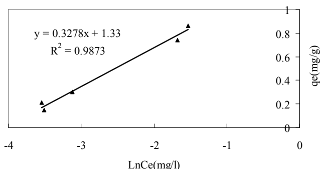
نمودار شماره ۸: ایزوترم تمکین برای جذب کروم در خاکستر استخوان (غلظت کروم ۱/۵ mg/l، دوز جاذب ۱۰۰ ml و ۰/۷ mg و pH=۳)
