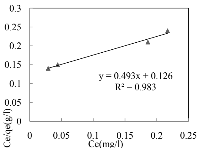
نمودار شماره ۷: ایزوترم Langmuir برای جذب کروم در خاکستر استخوان (غلظت کروم ۱/۵ mg/l، دوز جاذب ۱۰۰ ml و ۰/۷ mg و pH=۳)
