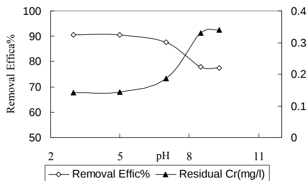
نمودار شماره ۲: تأثیر pH بر جذب کروم توسط خاکستر استخوان (غلظت کروم ۱/۵ mg/l، دوز جاذب ۰/۷ mg/۱۰۰ ml)
