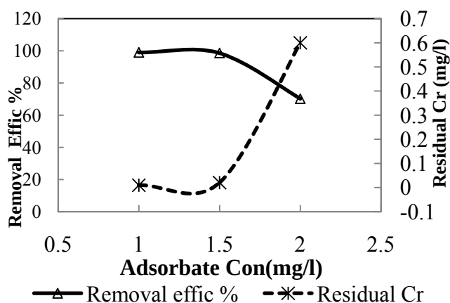
نمودار شماره ۳: تأثیر غلظت اولیه کروم بر جذب توسط خاکستر استخوان (pH=۳، دوز جاذب ۰/۷ mg/۱۰۰ ml)
