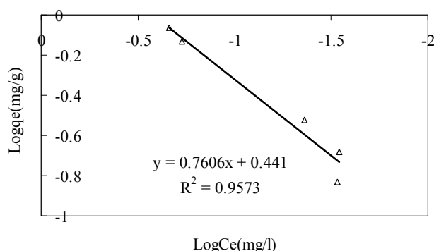
نمودار شماره ۶: ایزوترم Freundlich، برای جذب کروم در خاکستر استخوان (غلظت کروم ۱/۵ mg/l، دوز جاذب ۱۰۰ ml و ۰/۷ mg و pH=۳)
