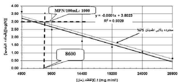
نمودار شماره ۱: رابطه میان C.T Value کل کلیفرم‌های باقی‌مانده پساب، در تماس با محلول کمپلکس هیدروژن پراکساید-یون نقره
