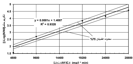
نمودار شماره ۲: رابطه میان C.T Value و کل کلیفرم‌های غیرفعال شده پساب، در تماس با محلول کمپلکس هیدروژن پراکساید-یون نقره
